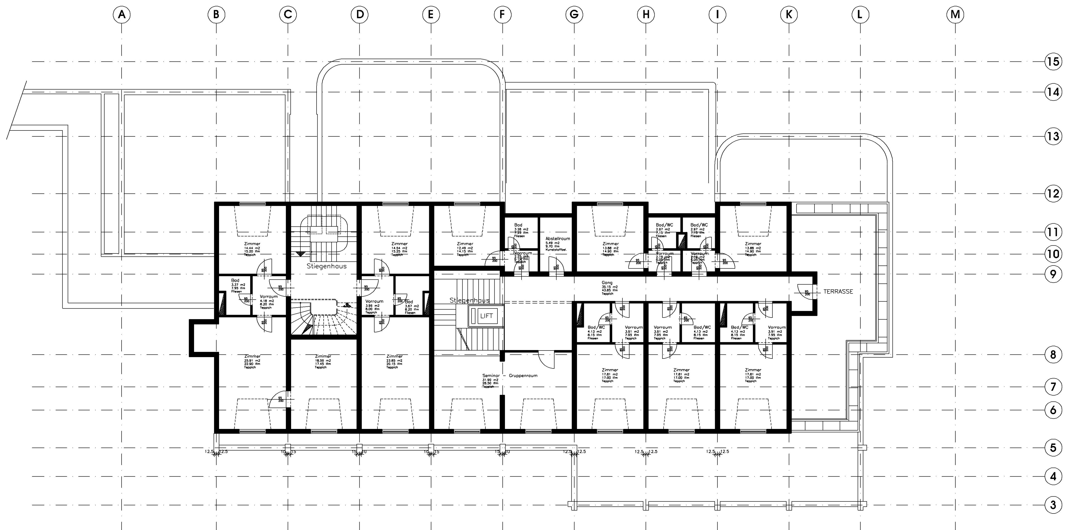
1. Obergeschoss
