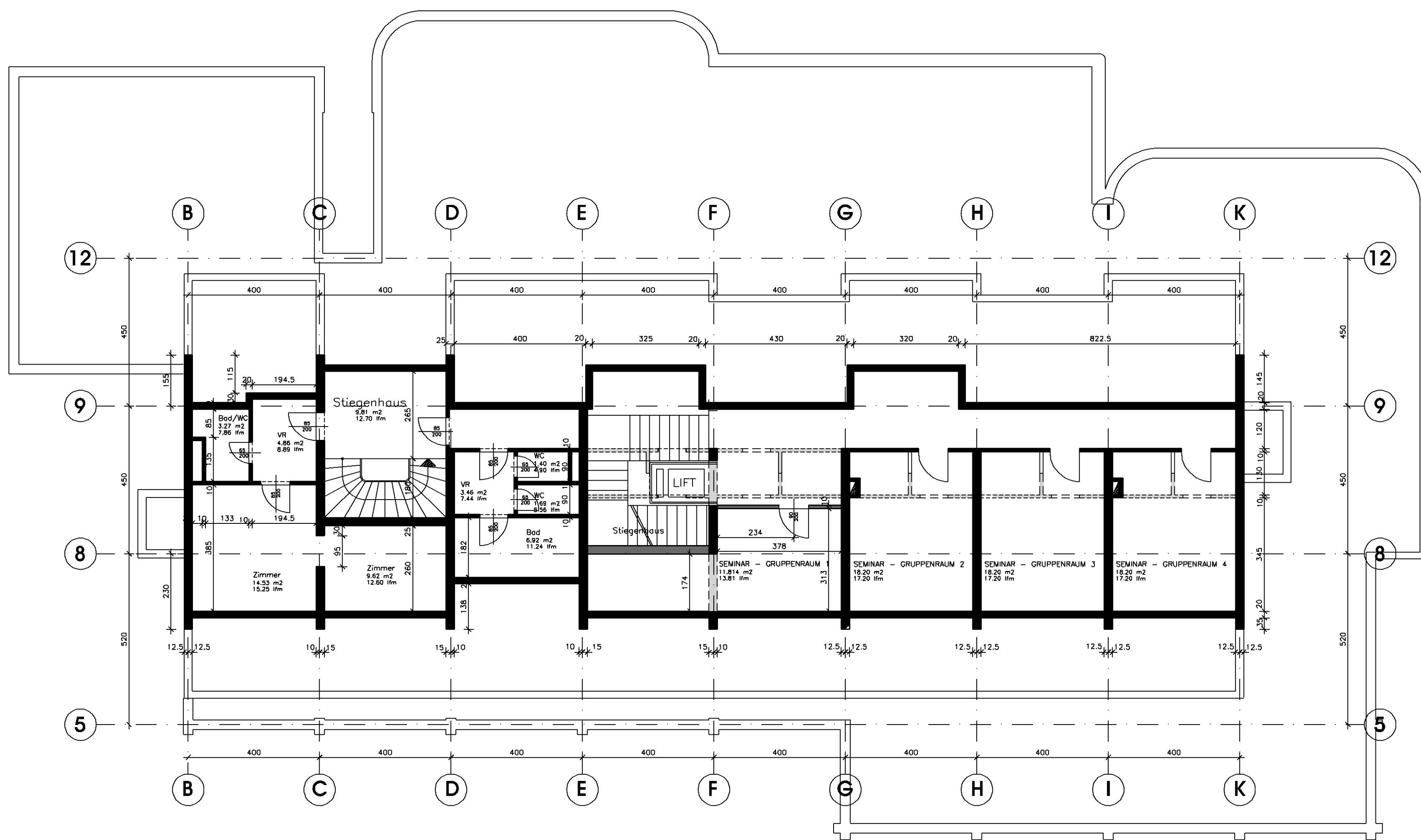
2. Obergeschoss
